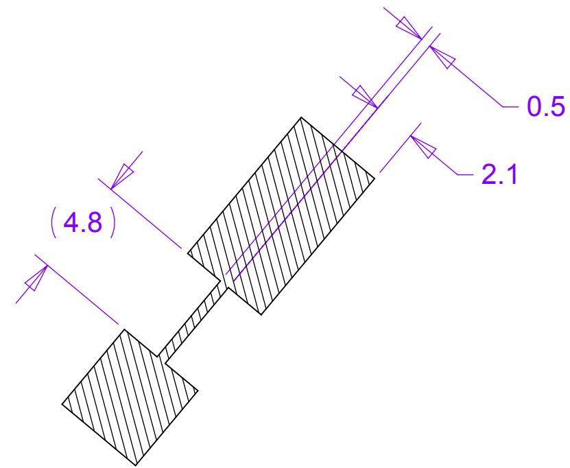
SECTION J-J VIEW TYP 3X
